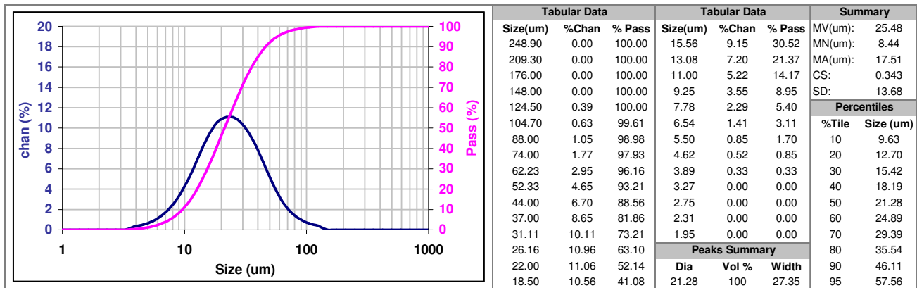
Fig. 6. Distribución Granulométrica
