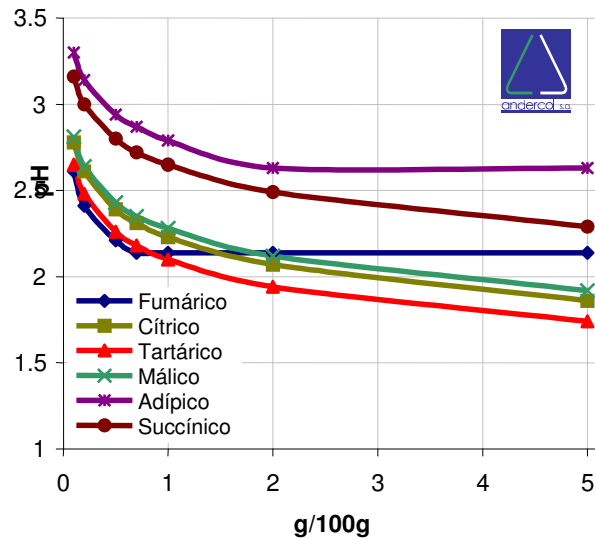
Fig. 3. pH para distintos acidulantes a 25 °C
