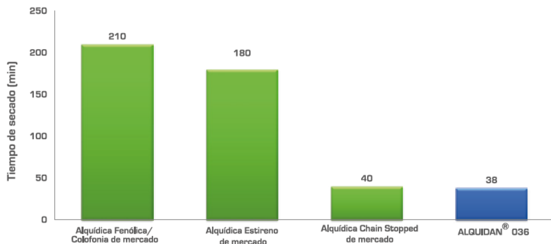
Figura 1. Tiempo de secado al manejo, Esmalte blanco con xileno en películas de 3 mils, ASTM D1640
