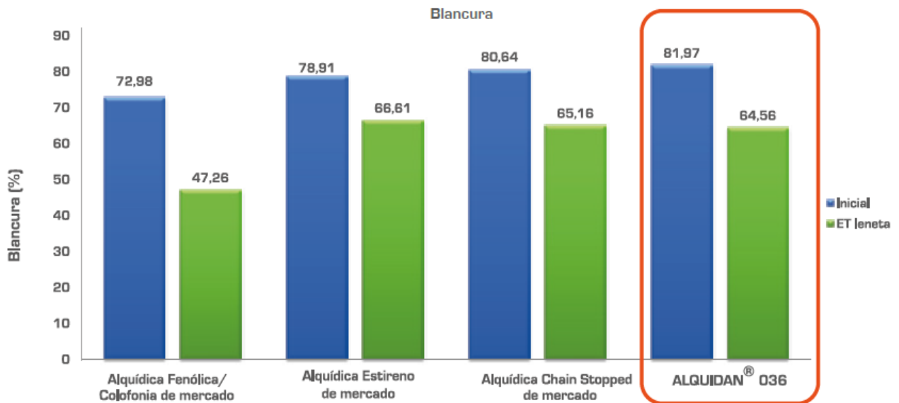
Figura 3. Blancura inicial y después de estabilidad térmica (ET) esmalte blanco con xileno
