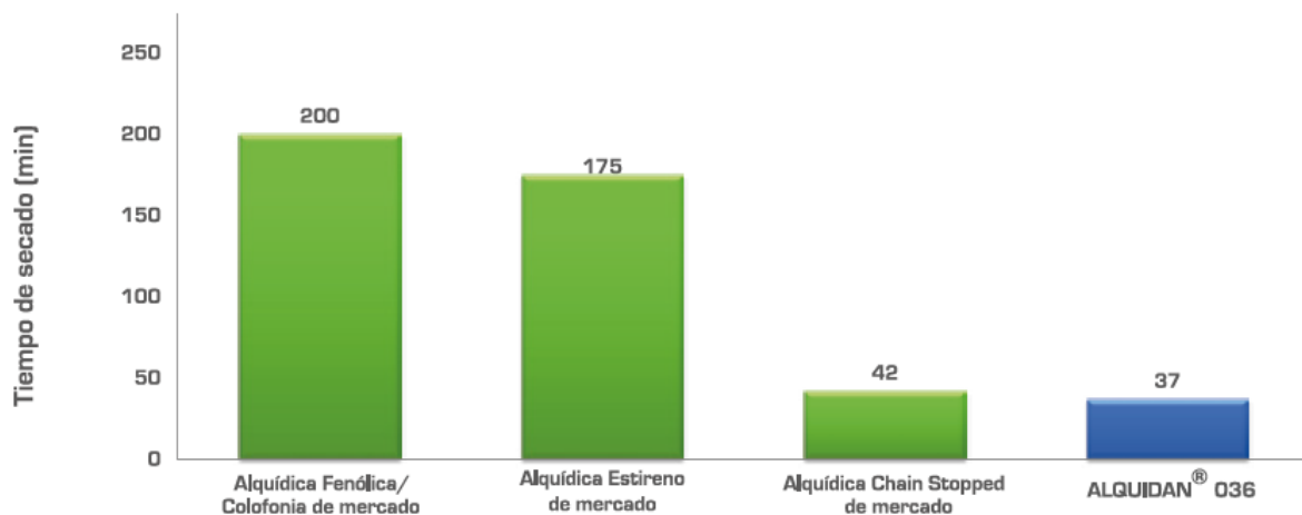
Figura 2. Tiempo de secado al manejo, Esmalte blanco con solvente alifático en películas de 3 mils, ASTM D1640
